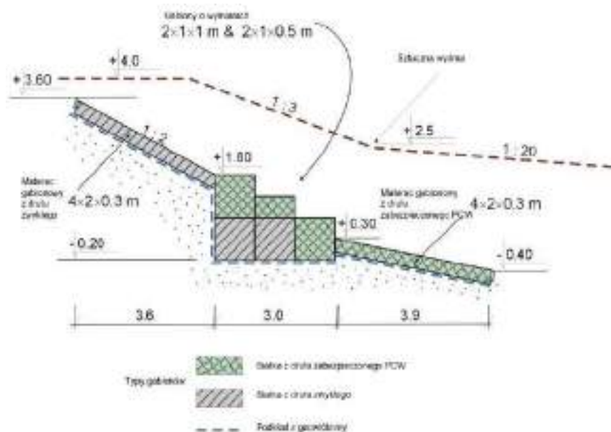
Rys. 1 Rysunek ideowy wydmę z rdzeniem gabionowym
