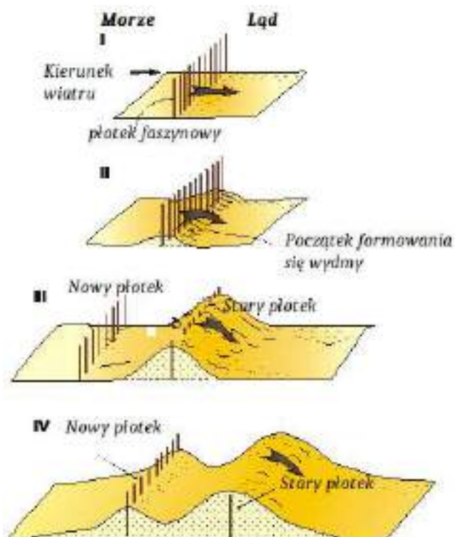
Rys. 1 Schemat powstawania wydym przez płotki faszynowe
