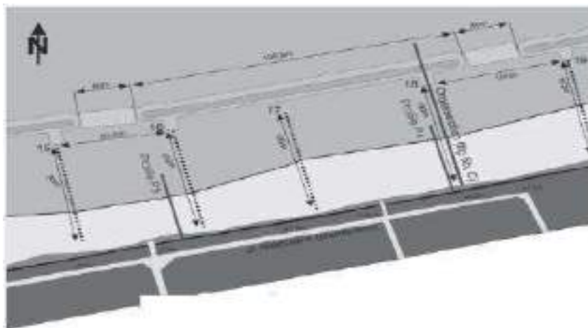
Rys. 1 Schemat rozmieszczenia progów podwodnych i ostróg w Kołobrzegu, źródło: Chuda i Kaczmarek 2018
