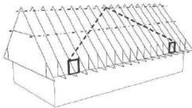
Schemat systemu stężenia wiatrowego z użyciem taśmy perforowanej
